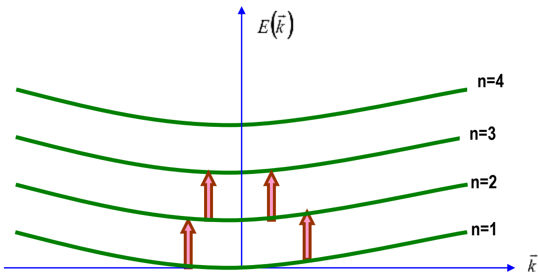
2-rasm. Oʻlchamli kvantlashgan tizimlarda tok tashuvchilarning vertikal (toʻgʻri) optikaviy oʻtishlari. Uzlüksiz egri chiziq tok tashuvchilarning energiyaviy spektrlari, n=1, 2, 3, 4 –oʻlchamli kvantlashgan energiyaviy spektrining tartib raqamlari. Tik vektorlar yordamida optikaviy oʻtishlar tasvirlangan.
